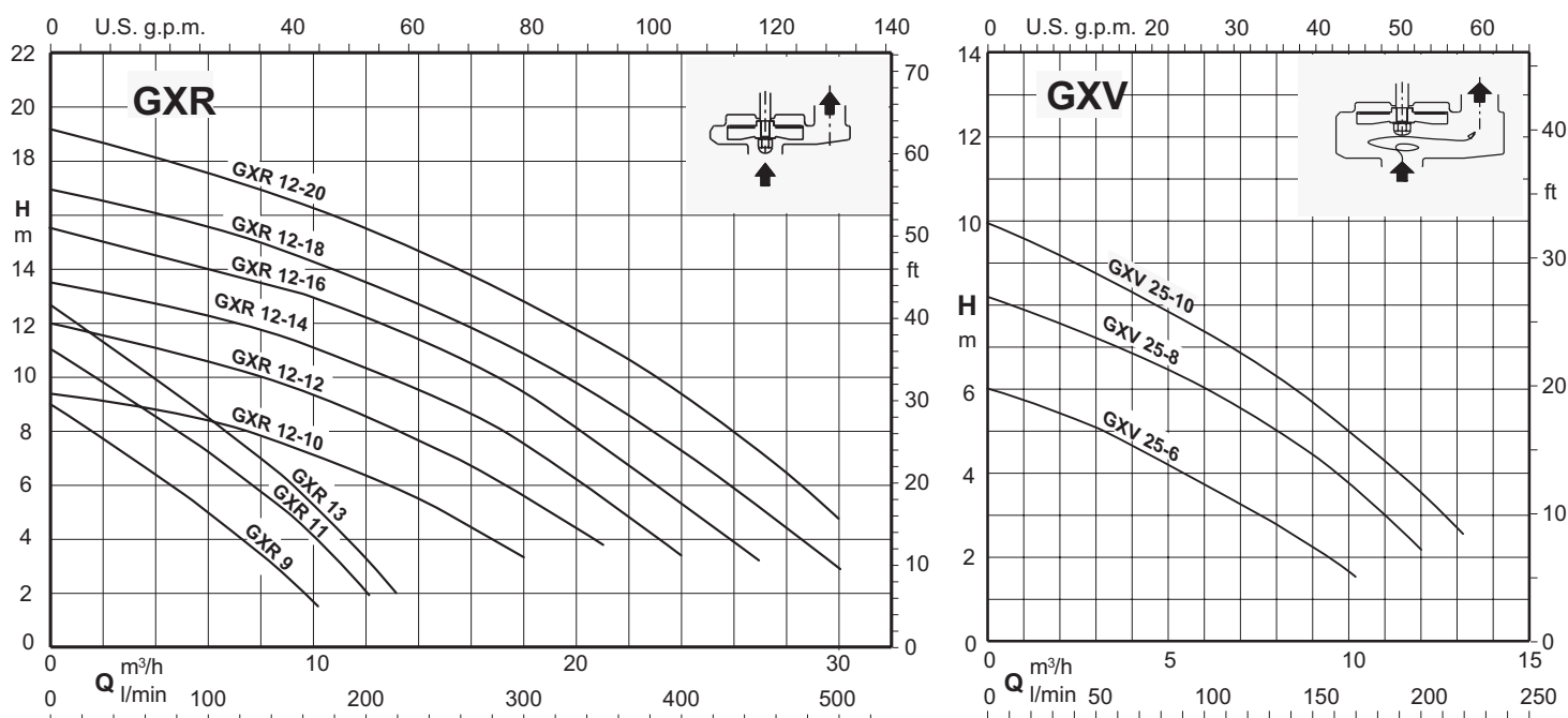
Graphique d'utilisation n \approx 2900 1/min
