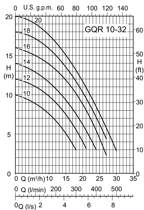
Graphique d'utilisation n \approx 2900 1/min
