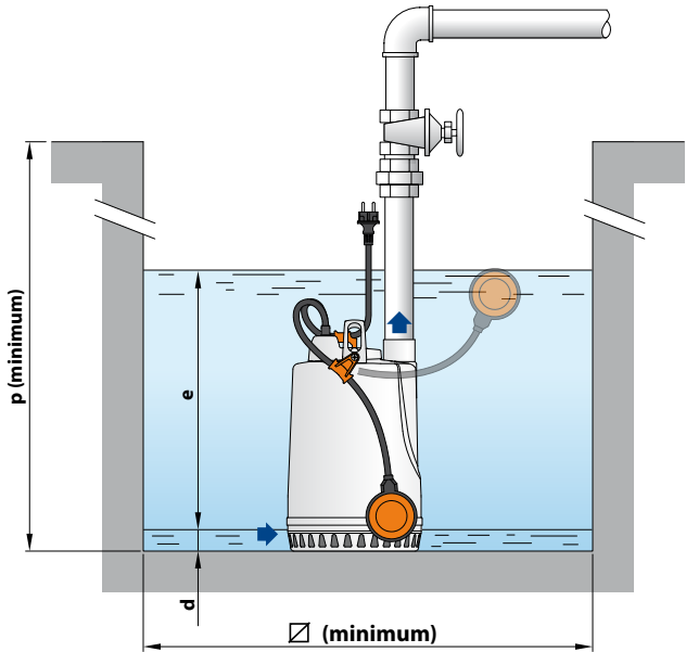
Installation typique
