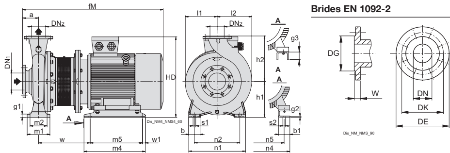
Brides EN 1092-2
