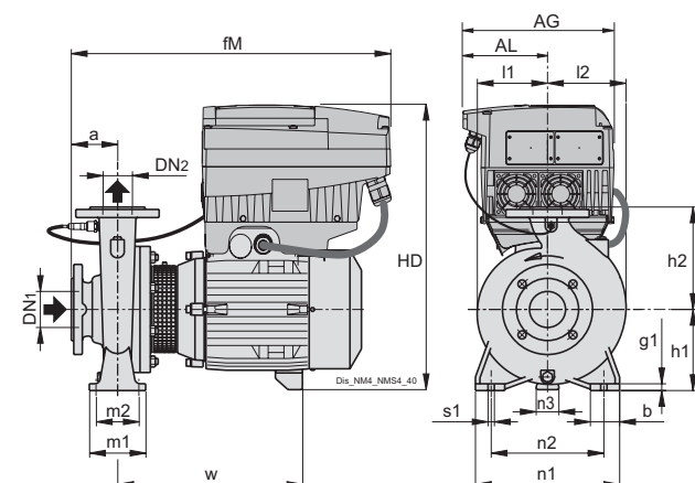
Brides EN 1092-2
