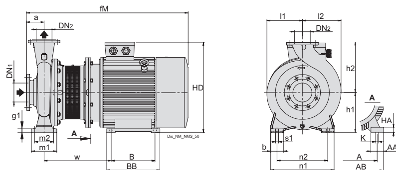
Brides EN 1092-2
