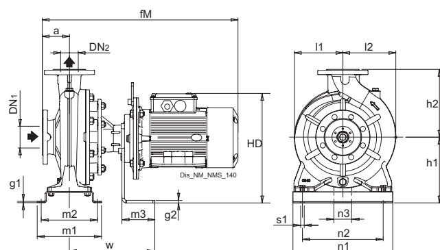
Brides EN 1092-2
