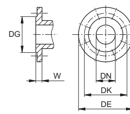
Brides EN 1092-2
