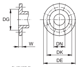
Brides EN 1092-2
