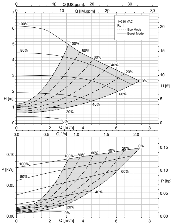
Calio 25-60 fonct. boucle ouverte, Eco-Mode
