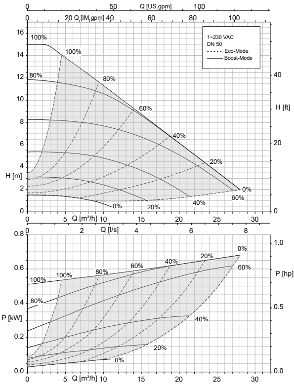
Calio 50-180 fonct. boucle ouverte, Eco-Mode
