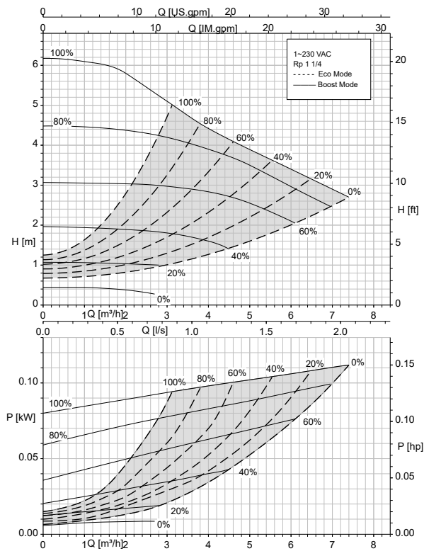
Calio 30-60 fonct. boucle ouverte, Eco-Mode
