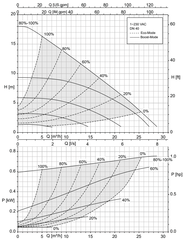
Calio 40-180 fonct. boucle ouverte, Eco-Mode
