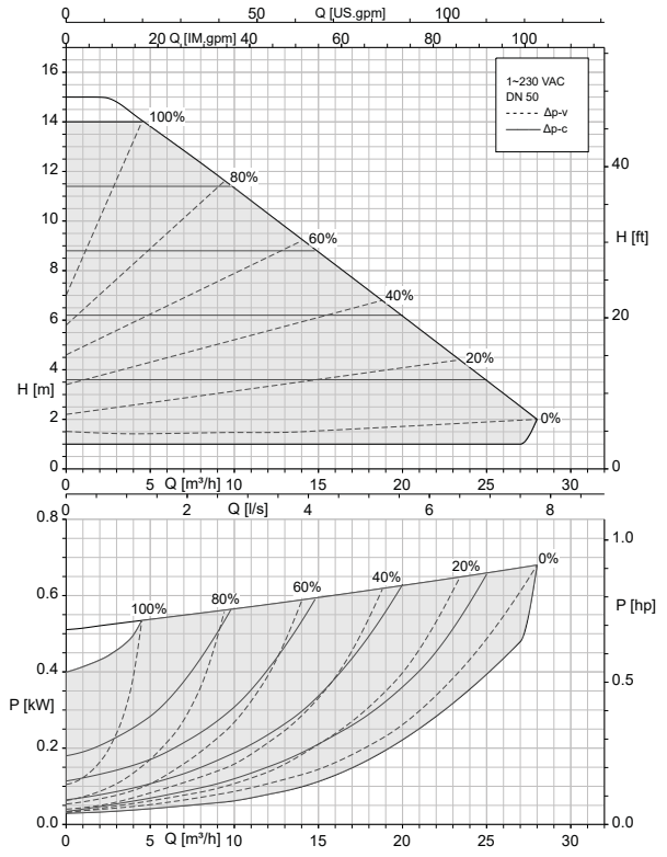
Calio 50-180 \Delta p -v, \Delta p -c
