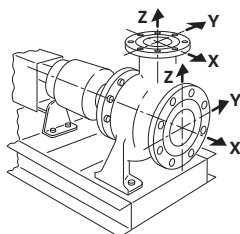
Fig. 15: Cas de charge 1A
